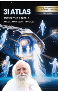
3i एटलस
